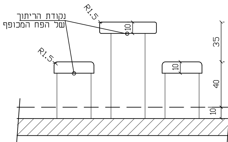
חתך ב-ב
