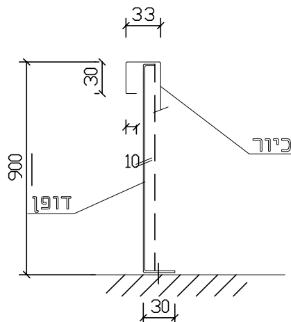
חתך א-א
