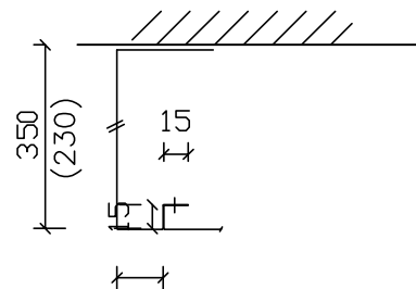
חתך ב-ב
